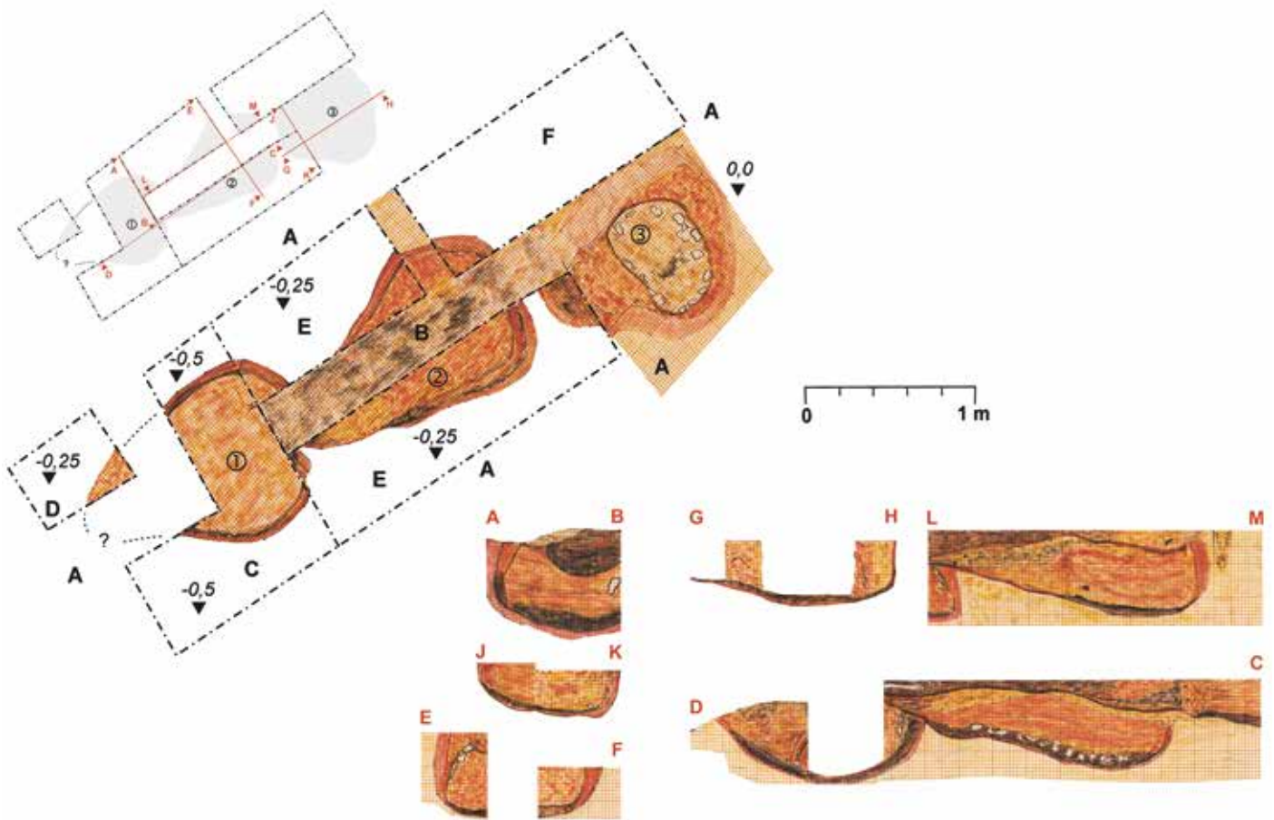
Abb. 2 Siegen, Hirschelsbachtal. Rennöfen des Schwarzwälder Typs der Ausgrabung K. Wilhelmi 1966. – (Graphik LWL-Archäologie für Westfalen / M. Zeiler auf Grundlage von K. Wilhelmi).
